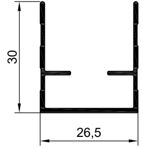
NO : 8112 AGIRLIK : 0.298 kg/m
