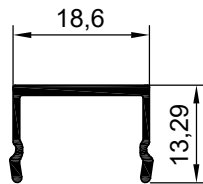
NO : 8008 AGIRLIK : 0.138 kg/m
