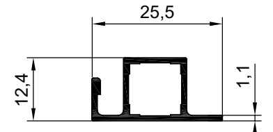
NO : 3505 AGIRLIK : 0.200 kg/m
