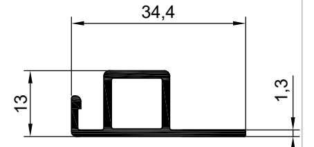
NO : 2861 AGIRLIK : 0.287 kg/m
