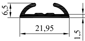
NO: 6756 AĞIRLIK:159 gr/m
