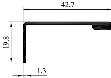
NO:6539 AĞIRLIK:275 gr/m
