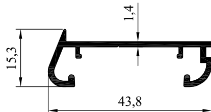
NO:6601 AĞIRLIK:320 gr/m
