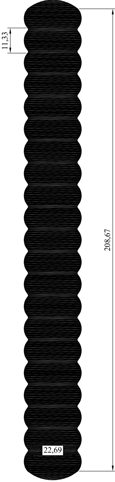
NO:7860 AĞIRLIK: 14208 gr/m
