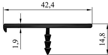
NO : 5823 AĞIRLIK : 292 gr/m
