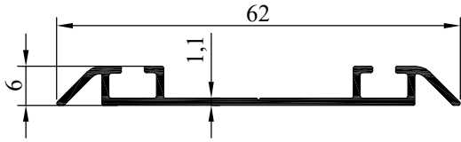
NO : 3474 AGIRLIK : 0.274 kg/m
