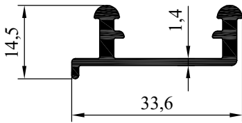
NO : 3954 AGIRLIK : 0.320 kg/m
