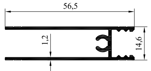
NO : 3475 AGIRLIK : 0.474 kg/m
