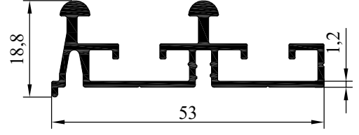
NO : 4819 AGIRLIK : 0.532 kg/m
