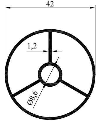
NO : 5104 AGIRLIK : 1.140 kg/m
