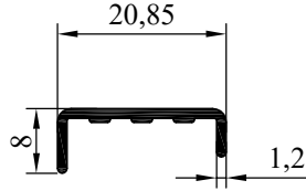
NO:6663 AĞIRLIK:111.6 gr/m
