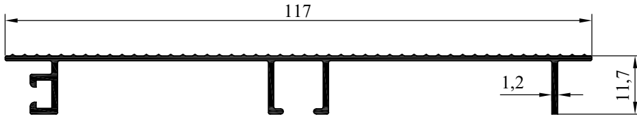
NO : 3525 AGIRLIK : 0.514 kg/m
