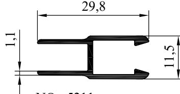
NO : 5211 AĞIRLIK : 0.234 kg/m
