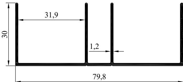
NO:7965 AĞIRLIK: 640 gr/m
