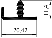
NO : 3685 AGIRLIK : 0.191 kg/m
