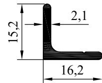
NO: 7408 AĞIRLIK:168 gr/m
