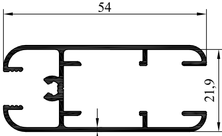
NO:6828 AĞIRLIK: 570 gr/m
