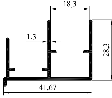
NO : 4817 AGIRLIK : 0.444 kg/m
