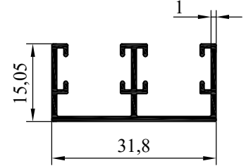
NO : 5213 AGIRLIK : 0.266 kg/m
