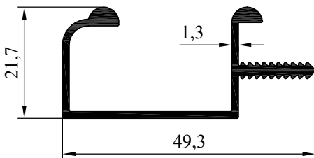
NO : 5123 AĞIRLIK : 0.437 kg/m
