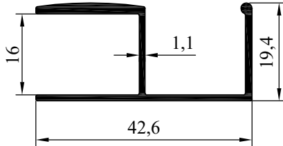
NO : 3402 AĞIRLIK : 0.366 kg/m
