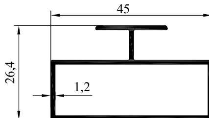
NO : 4275 AĞIRLIK : 0.480 kg/m
