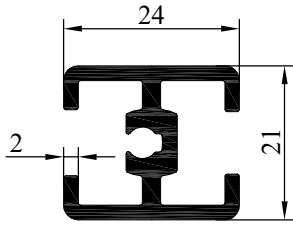
NO : 4249 AĞIRLIK : 0.513 kg/m
