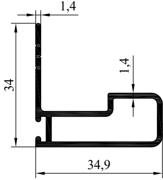
NO : 5735 AĞIRLIK : 447 gr/m
