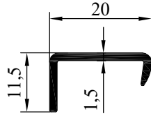
NO : 3404 AGIRLIK : 0.135 kg/m
