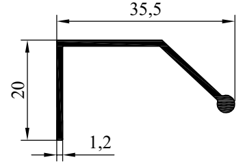
NO: 6693 AĞIRLIK: 207 gr/m
