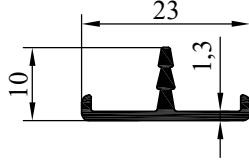
NO : 763 AGIRLIK : 0.136 kg/m
