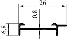
NO : 2056 AGIRLIK : 0.090 kg/m
