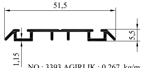
NO : 3393 AGIRLIK : 0.267 kg/m
