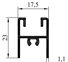
NO:6830 AĞIRLIK: 266 gr/m
