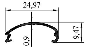
NO:7721 AGIRLIK: 103 gr/m
