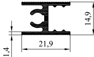
NO : 5727 AĞIRLIK : 296 gr/m
