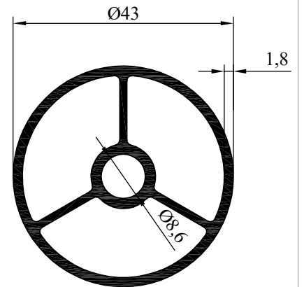
NO : 6030 AGIRLIK : 968 gr/m
