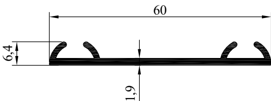
NO : 3398 AGIRLIK : 0.396 kg/m
