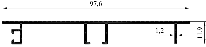
NO : 4421 AGIRLIK : 0.481 kg/m
