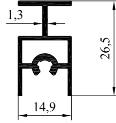
NO:7512 AĞIRLIK: 286 gr/m
