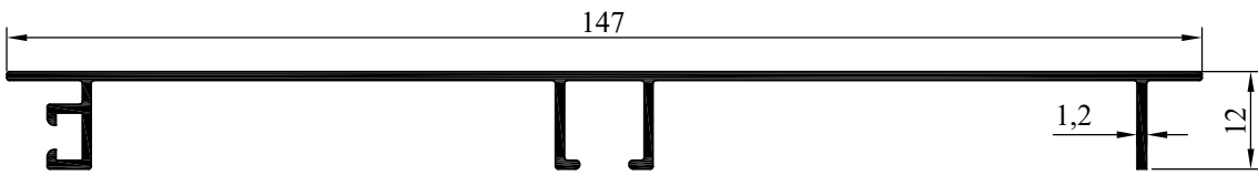
NO : 3528 AGIRLIK : 0.613 kg/m
