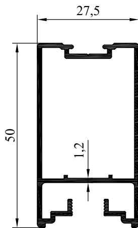
NO:6835 AĞIRLIK: 575 gr/m
