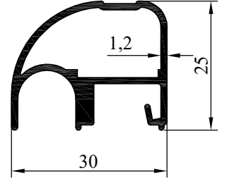
NO.6749 AĞIRLIK: 421 gr/m
