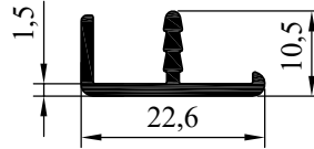
NO : 4003 AGIRLIK : 0.172 kg/m
