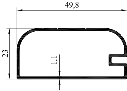
NO : 4285 AĞIRLIK : 0.435 kg/m
