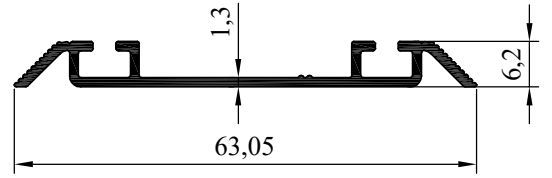
NO : 5726 AĞIRLIK : 325 gr/m
