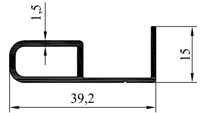
NO : 6065 AĞIRLIK : 322 gr/m
