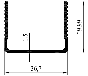
NO:7747 AĞIRLIK: 411 gr/m
