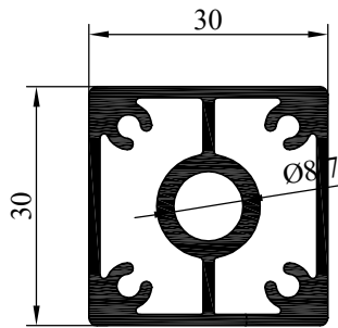
NO : 4027 AGIRLIK : 0.934 kg/m
