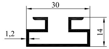
NO : 6321 AĞIRLIK : 275 gr/m
