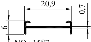
NO : 1587 AGIRLIK : 0.066 kg/m
