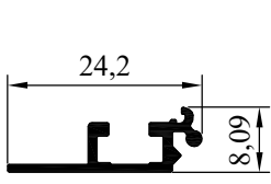
NO : 3236 AGIRLIK : 0.130 kg/m
