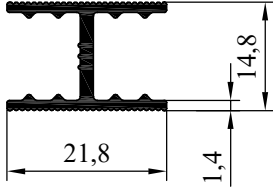
NO : 5729 AĞIRLIK : 230 gr/m
