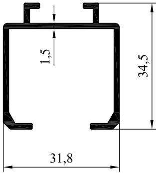
NO:7514 AĞIRLIK:478 gr/m
