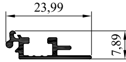
NO:7722 AGIRLIK: 130 gr/m
