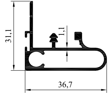
NO : 4818 AĞIRLIK : 0.457 kg/m
