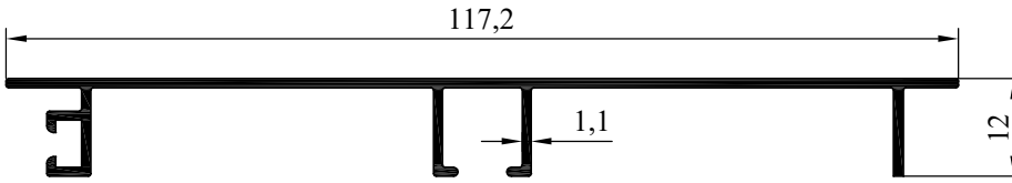
NO : 3526 AGIRLIK : 0.524 kg/m
