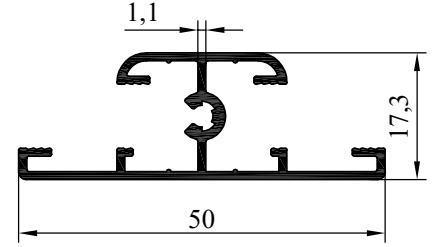
NO:6554 AĞIRLIK:385 gr/m
