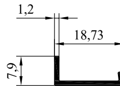
NO : 3776 AGIRLIK : 0.090 kg/m
