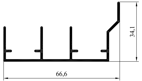
NO:7958 AĞIRLIK: 577 gr/m
