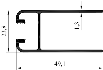
NO : 5694 AĞIRLIK : 489 gr/m
