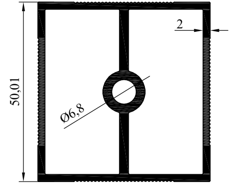
NO : 4685 AGIRLIK : 1.398 kg/m
