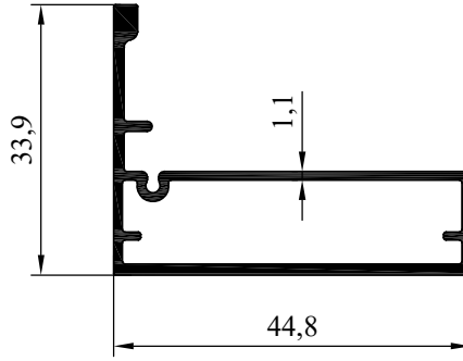
NO:7946 AĞIRLIK: 497 gr/m
