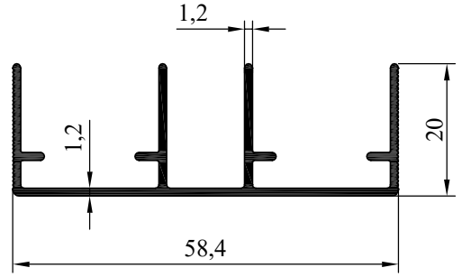
NO : 5642 AĞIRLIK: 470 gr/m
