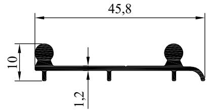
NO : 3403 AGIRLIK : 0.305 kg/m
