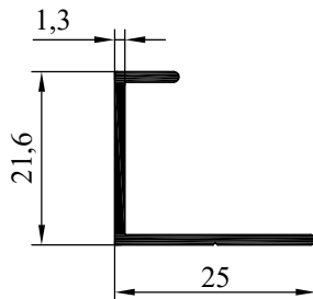
NO:6538 AĞIRLIK: 182 gr/m
