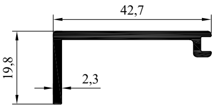
NO:6451 AĞIRLIK:397 gr/m
