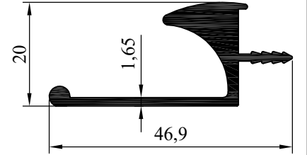
NO:7299 AĞIRLIK:540 gr/m
