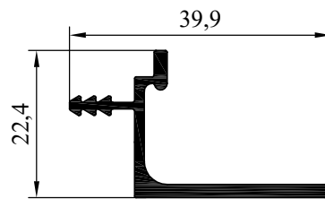
NO : 4031 AĞIRLIK : 0.318 kg/m
