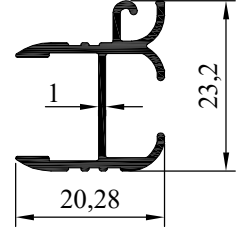
NO : 4837 AGIRLIK : 0.239 kg/m
