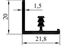
NO : 3838 AGIRLIK : 0.241 kg/m
