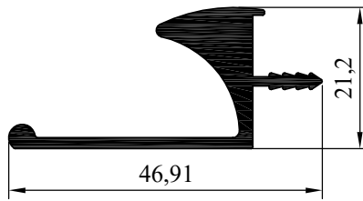
NO : 4616 AĞIRLIK : 0.575 kg/m
