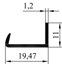
NO : 4041 AGIRLIK : 0.110 kg/m
