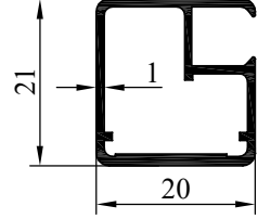
NO : 3807 AĞIRLIK : 0.261 kg/m
