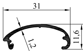
NO : 4213 AGIRLIK : 0.165 kg/m
