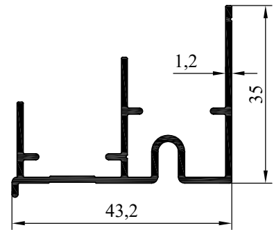
NO:8108 AĞIRLIK: 467 gr/m
