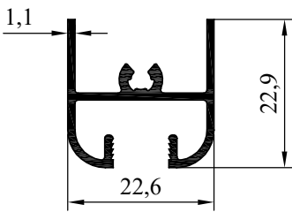
NO:6642 AĞIRLIK:285 gr/m
