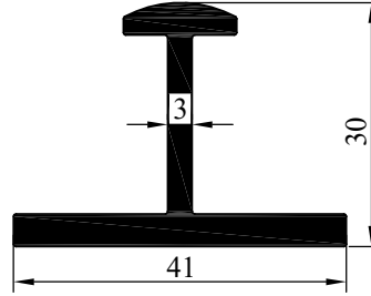
NO:8050 AĞIRLIK: 751 gr/m
