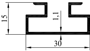
NO:7983 AĞIRLIK: 257 gr/m
