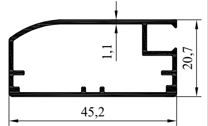
NO : 3559 AGIRLIK : 0.437 kg/m
