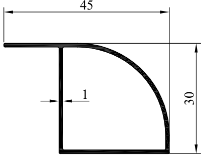
NO:2722 AĞIRLIK : 0.325 kg/m
