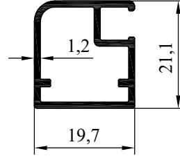
NO:7495 AĞIRLIK: 286 gr/m
