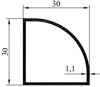
NO : 2676 AĞIRLIK : 0.312 kg/m
