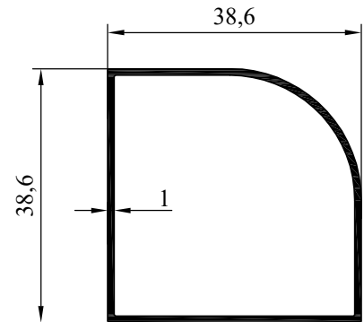
NO : 5415 AĞIRLIK :0.384 kg/m
