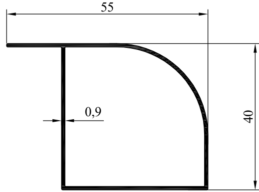
NO : 5431 AGIRLIK : 0.392 kg/m
