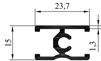
NO:6751 AĞIRLIK: 295 gr/m
