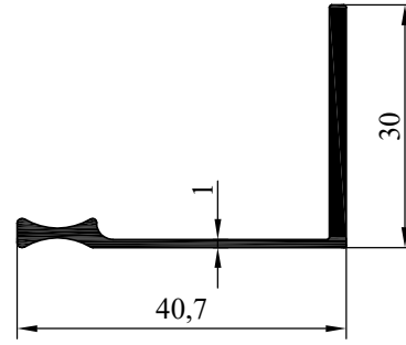
NO:6777 AĞIRLIK: 0.308 gr/m
