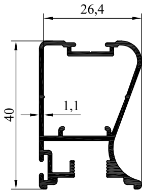
NO:6831 AĞIRLIK:516 gr/m
