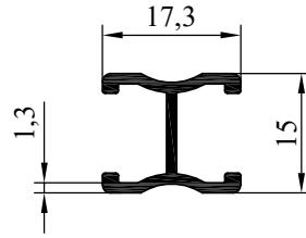
NO : 3540 AGIRLIK : 0.183 kg/m
