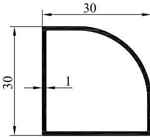
NO : 3458 AĞIRLIK : 0.290 kg/m
