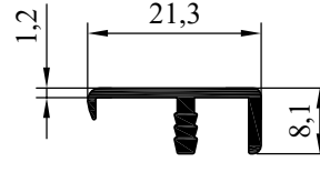
NO:6665 AĞIRLIK:144.7 gr/m
