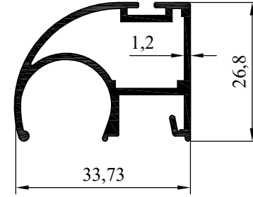
NO:6755 AĞIRLIK:463 gr/m
