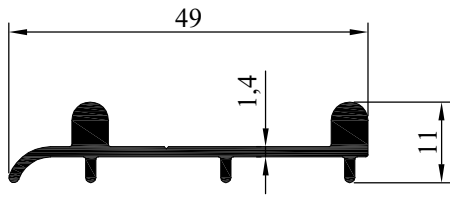
NO : 3392 AGIRLIK : 0.379 kg/m
