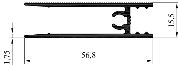
NO : 5728 AĞIRLIK : 605 gr/m
