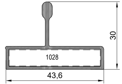
1725 0,507 kg/mt
