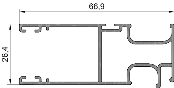
13-09986 0,741 kg/mt
