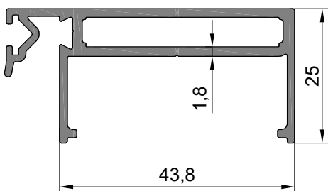
ASM41T-41 0,707 kg/mt
