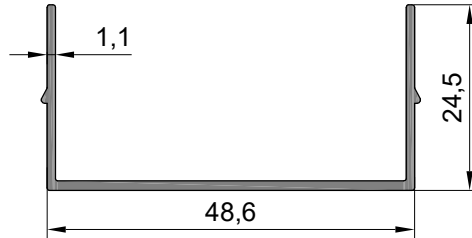
ASM41T-64 0,302 kg/mt
