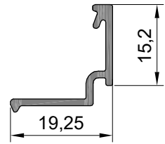
ASM10-04 0,157 kg/mt
