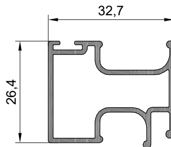
18677 0,468 kg/mt
