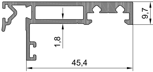
ASM41T-42 0,734 kg/mt
