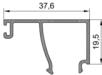
ASM41T-38 0,346 kg/mt
