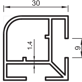
No : 2704 Dikme 1,100 kg/m
