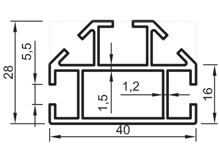
No : 2633 Dikme 0,660 kg/m
