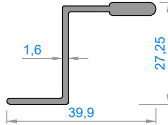
1768 - 0,338 kg/m
