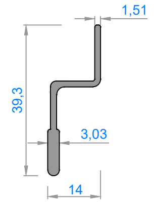
1142 - 0,257 kg/m
