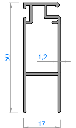
4867 - 0,470 kg/m
