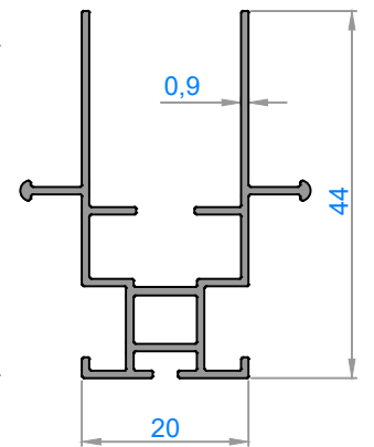
4474 - 0,395 kg/m
