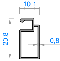
1727 - 0,143 kg/m
