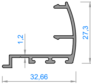
3015 - 0,300 kg/m
