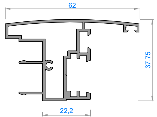
3008 - 0,805 kg/m
