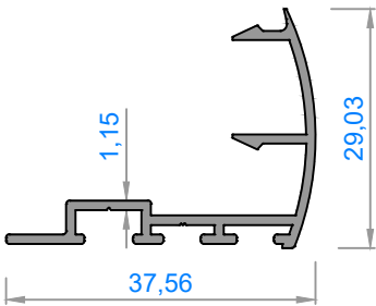
1333 - 0,305 kg/m
