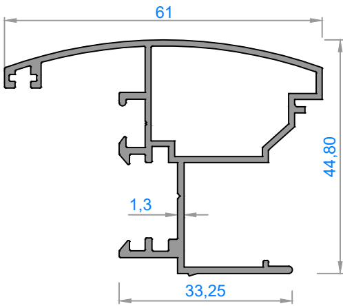
1305 - 0,725 kg/m
