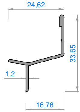
1330 - 0,182 kg/m
