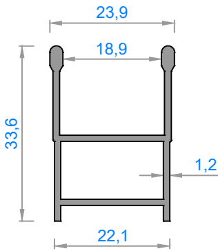
3020 - 0,385 kg/m
