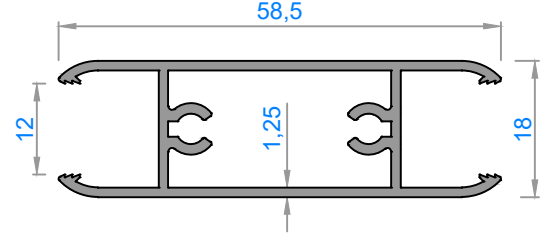
3058 - 0,605 kg/m
