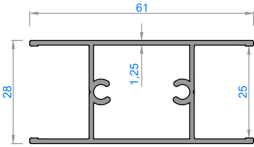
1313 - 0,665 kg/m
