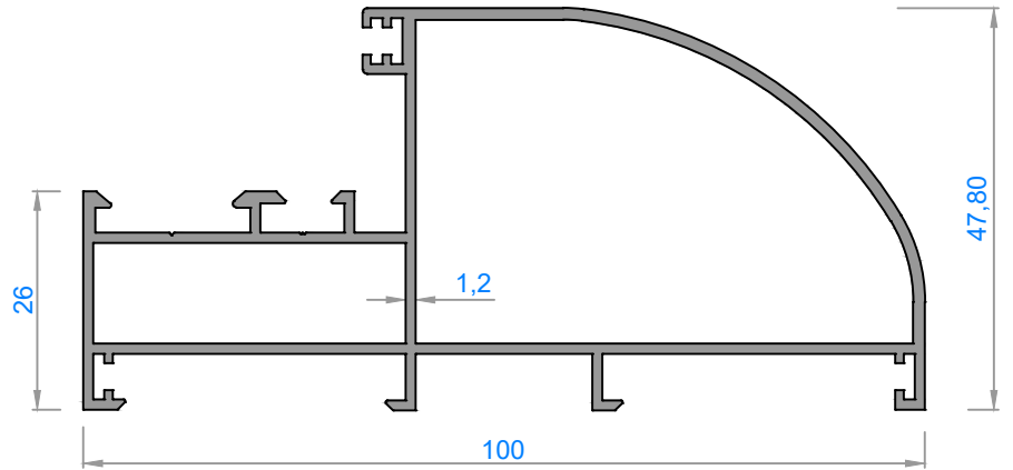
1325 - 1,190 kg/m
