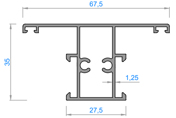
3006 - 0,735 kg/m
