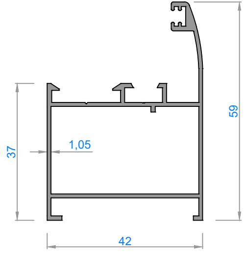
1303 - 0,630 kg/m
