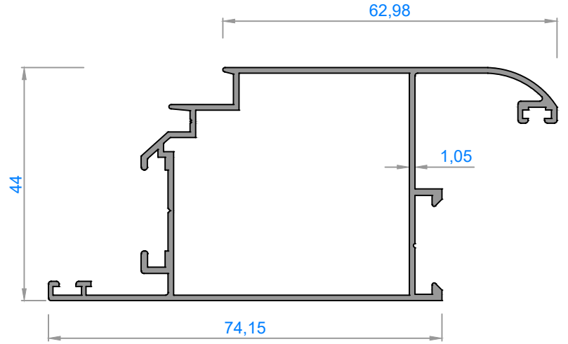
1308 - 0,840 kg/m
