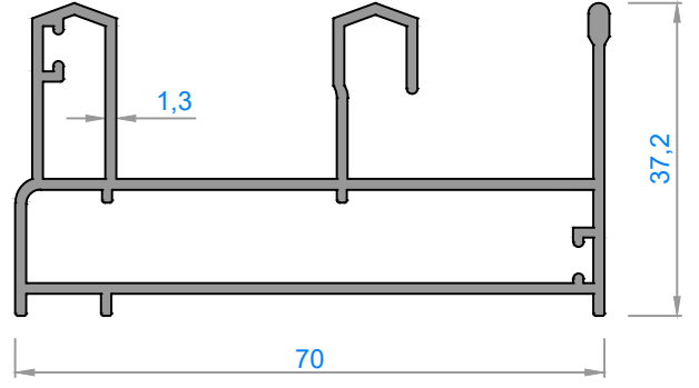
3016 - 1,014 kg/m
