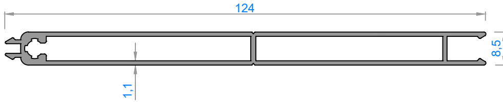
3035 - 0,840 kg/m
