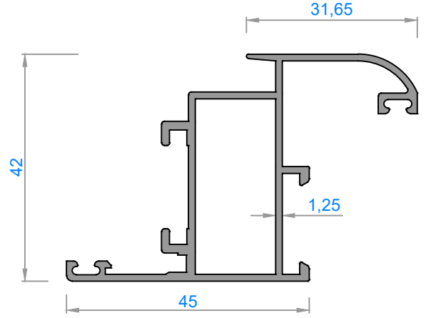
2988 - 0,745 kg/m
