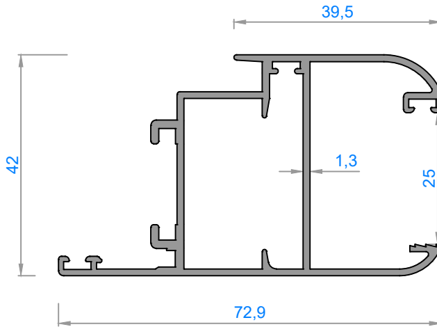
3057 - 0,935 kg/m
