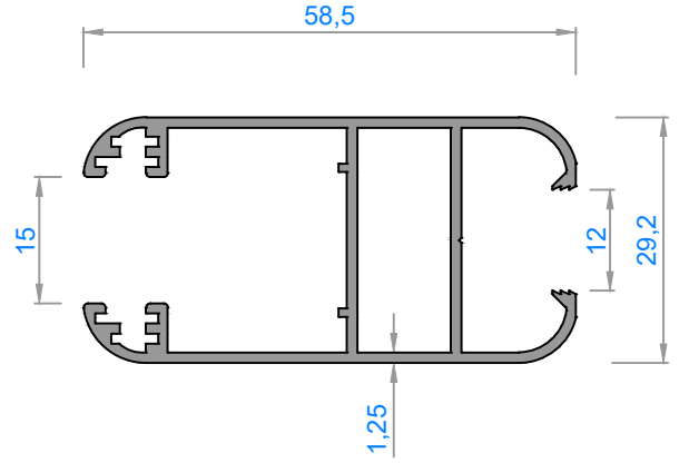
3014 - 0,723 kg/m
