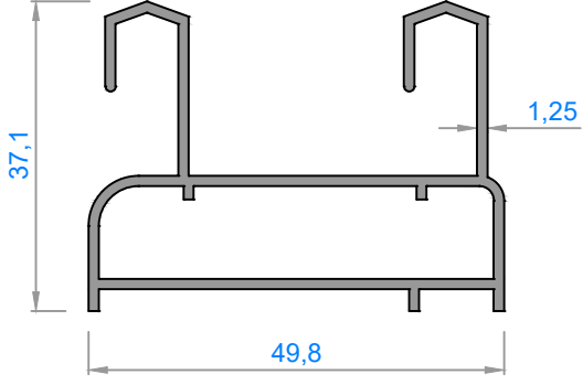
3013 - 0,684 kg/m
