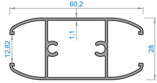
1314 - 0,658 kg/m
