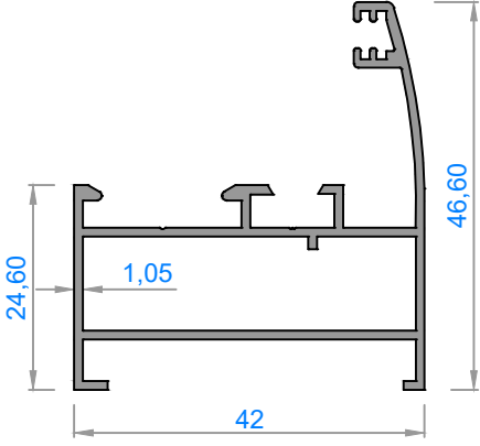
1304 - 0,550 kg/m
