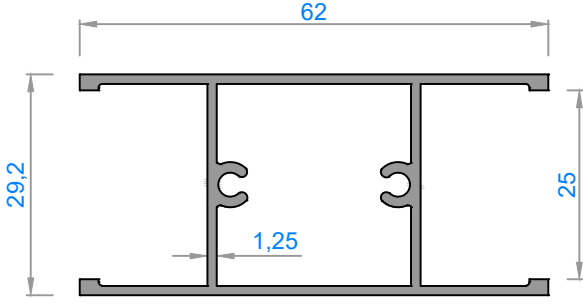
3116 - 0,695 kg/m
