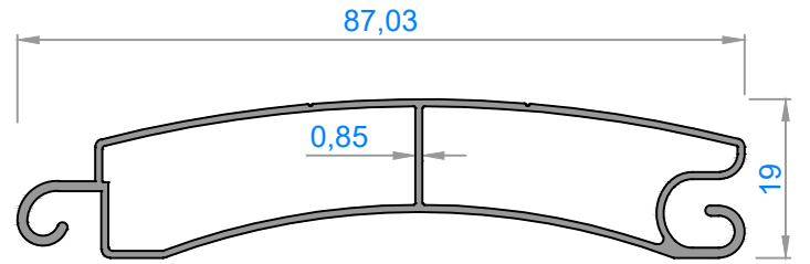
1507 - 0,555 kg/m
