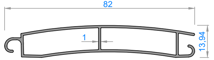
3254 - 0,532 kg/m
