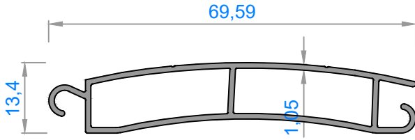
2455 - 0,480 kg/m
