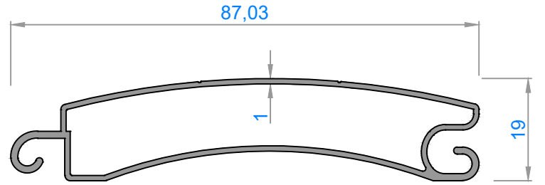
1505 - 0,607 kg/m
