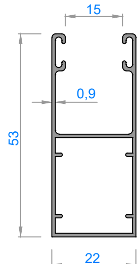
3059 - 0,420 kg/m
