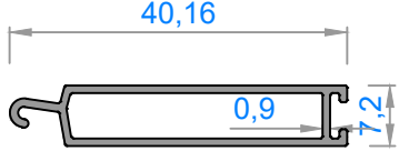
3626 - 0,222 kg/m
