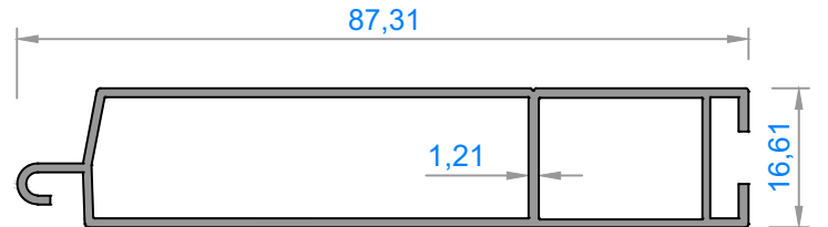
1503 - 0,642 kg/m
