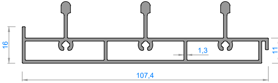
6202 - 1,305 kg/m
