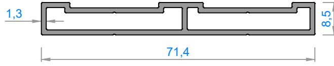
6201 - 0,585 kg/m
