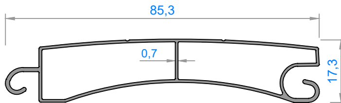
4227 - 0,484 kg/m
