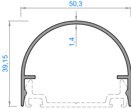
Sistem Kodu : FC50-6023 Ağırlık (kg/mt): 0,450
