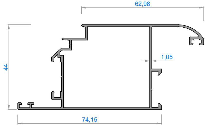
1308 - 0,840 kg/m
