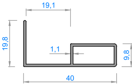
4406 - 0,278 kg/m
