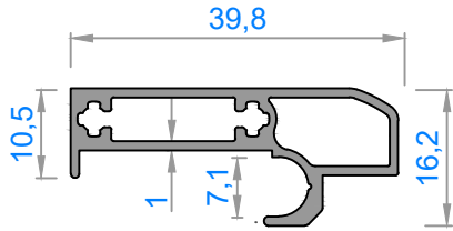
3123 - 0,368 kg/m
