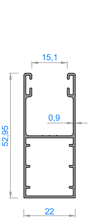
2255 - 0,430 kg/m
