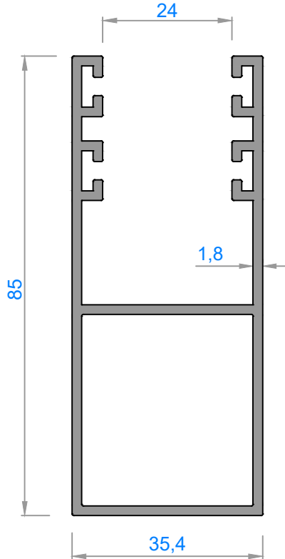
1501- 1,370 kg/m
