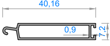
3626 - 0,222 kg/m
