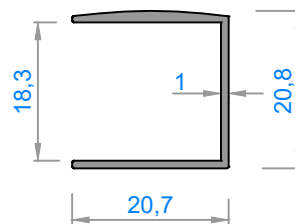
4429 - 0,176 kg/m
