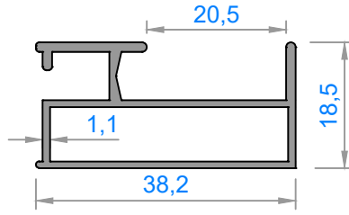
4396 - 0,381 kg/m
