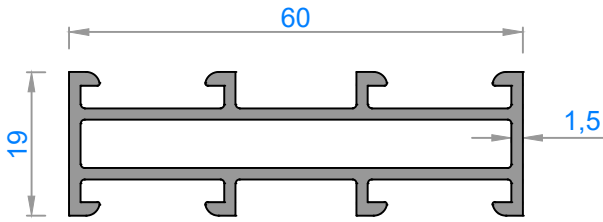
1150 - 0,784 kg/m
