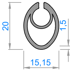
1192 - 0,263 kg/m
