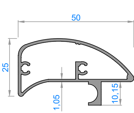
1879 - 0,569 kg/m
