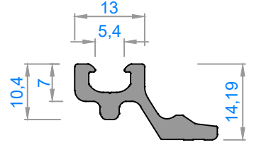
Sistem Kodu : FC50-6028 Ağırlık (kg/mt): 0,145
