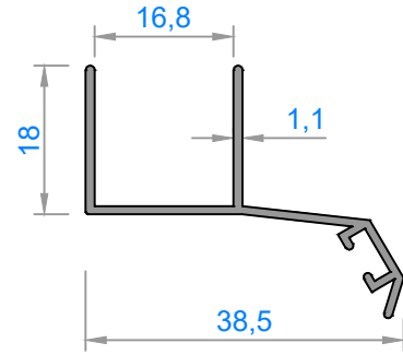
4403 - 0,250 kg/m
