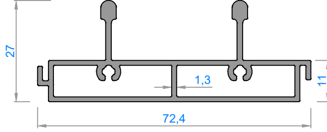
6200 - 0,880 kg/m
