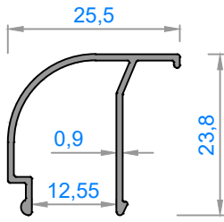
3463 - 0,173 kg/m
