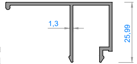
* 4503 - 0,361 kg/m
