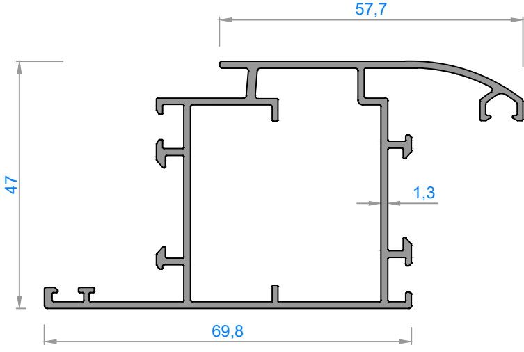
5388 - 1,064 kg/m
