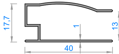
3126 - 0,276 kg/m
