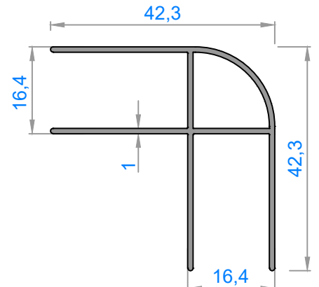
1226 - 0,431 kg/m STOK BOYU : 550 cm
