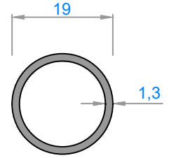
2140 - 0,196kg/m
