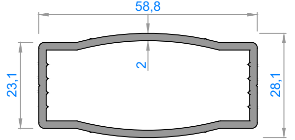
1195 - 0,855 kg/m
