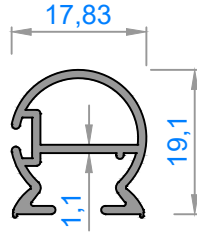
1284 - 0,242 kg/m STOK BOYU : 540 cm
