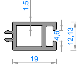
Sistem Kodu : FC50-6026 Ağırlık (kg/mt): 0,315
