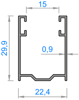
3884 - 0,245 kg/m
