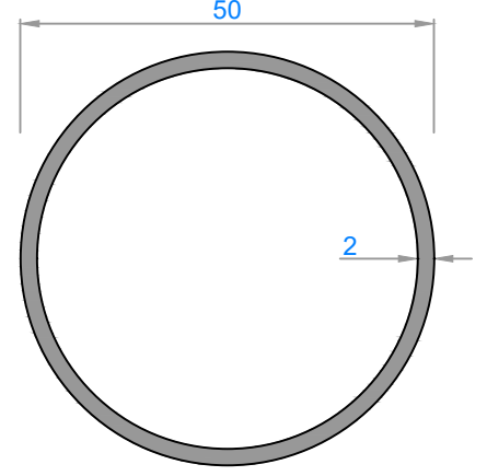
1007 - 0,819 kg/m
