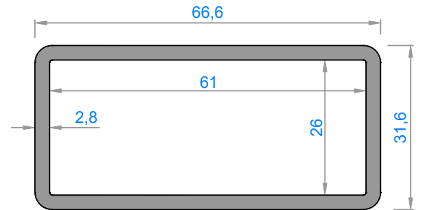
4481- 1,380 kg/m
