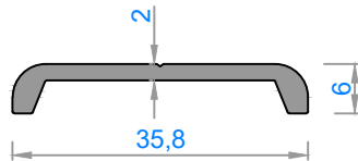
4536- 0,245 kg/m
