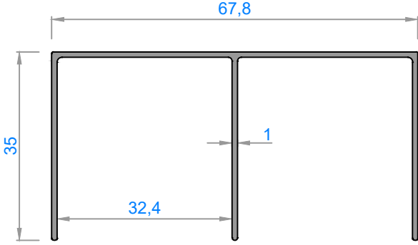
4051 - 0,460 kg/m
