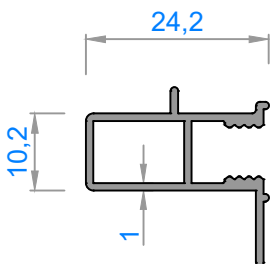
1473 - 0,236 kg/m
