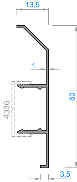
3918 - 0,272 kg/m
