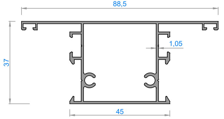
1306 - 0,810 kg/m
