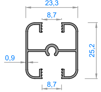
4050 - 0,285 kg/m
