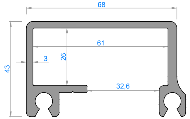
4295 - 1,758 kg/m
