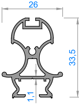
1288 - 0,455 kg/m STOK BOYU : 540 cm
