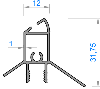
4397 - 0,338 kg/m
