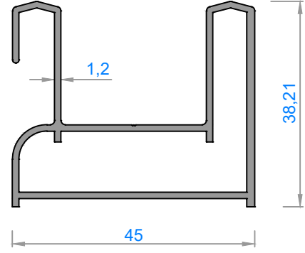
1317 - 0,685 kg/m
