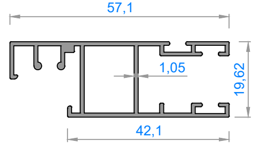
1770 - 0,304 kg/m
