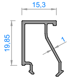
Sistem Kodu : 6168 Ağırlık (kg/mt): 0,222
