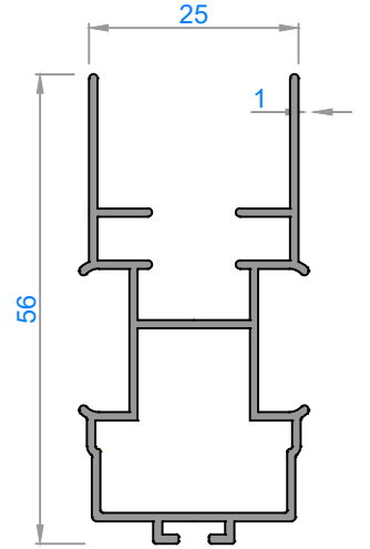
4474 - 0,395 kg/m
