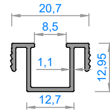
6208 - 0,180 kg/m
