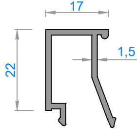
1152 - 0,298 kg/m
