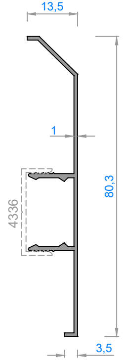
3919 - 0,323 kg/m
