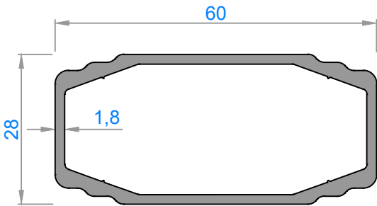
1360 - 0,904 kg/m
