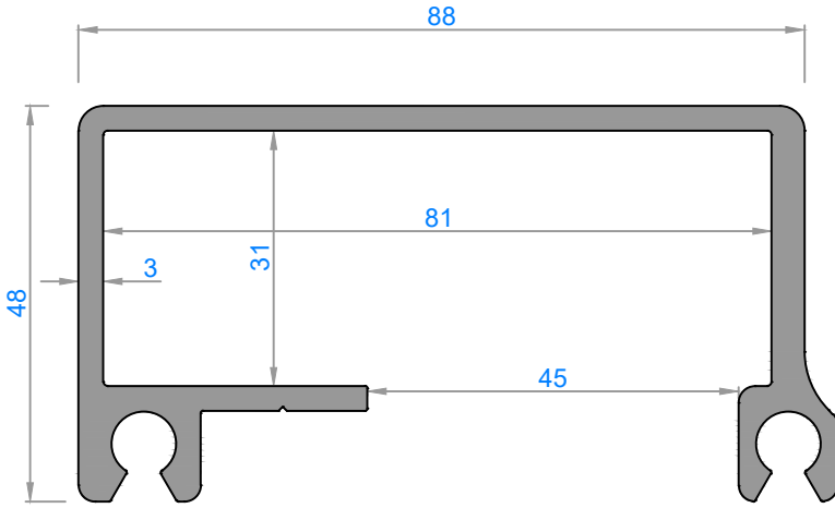
4296 - 2,077 kg/m
