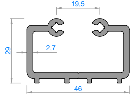
Sistem Kodu : FC50-6032 Ağırlık (kg/mt): 1,670
