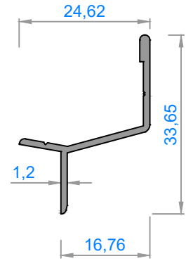
1330 - 0,182 kg/m
