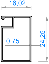
1725 - 0,176 kg/m
