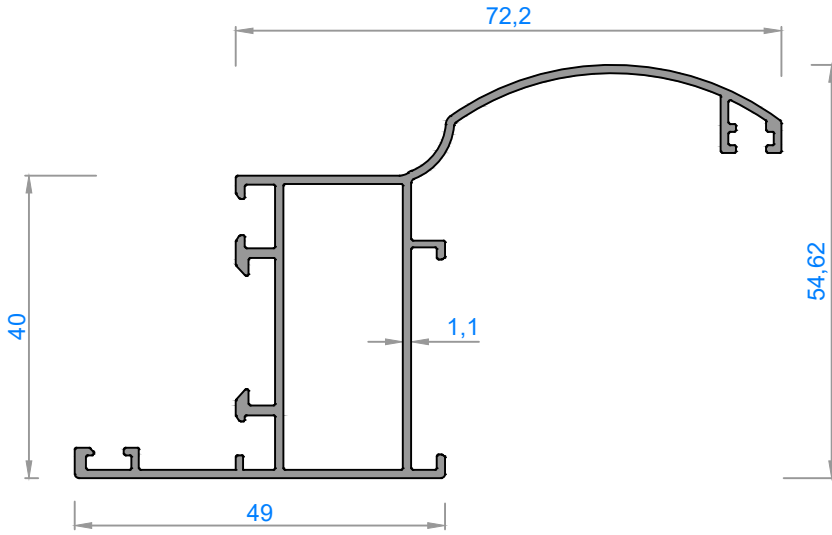
5387 - 0,770 kg/m
