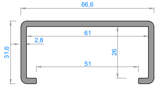
4293 - 0,997 kg/m
