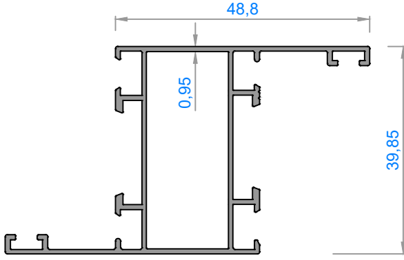
4092 - 0,564 kg/m
