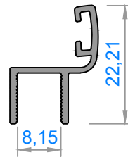
4166 - 0,171 kg/m
