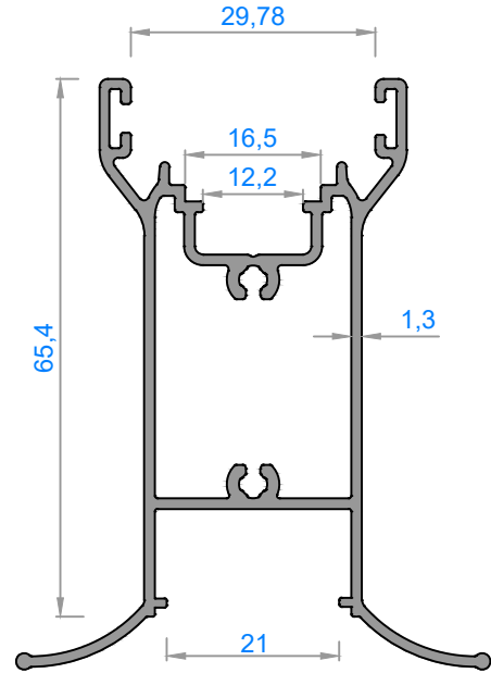
6209 - 1,005 kg/m
