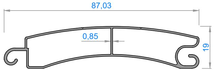
1507 - 0,555 kg/m
