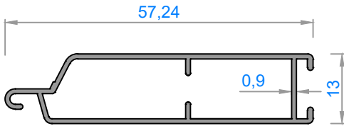
3891 - 0,347 kg/m
