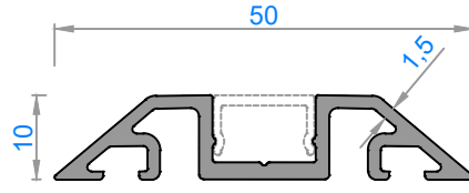
Sistem Kodu : FC50-6041 Ağırlık (kg/mt): 0,413 Statik J_x (cm 4 ): 1,50 J_y (cm 4 ): 2,86
