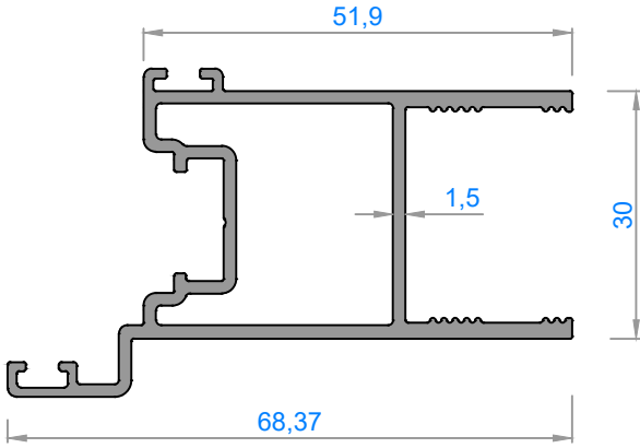
5983 - 0,936 kg/m
