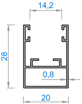
3625 - 0,265 kg/m
