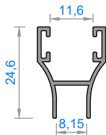
4825 - 0,210 kg/m
