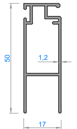
4867 - 0,470 kg/m
