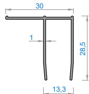
4818 - 0,230 kg/m
