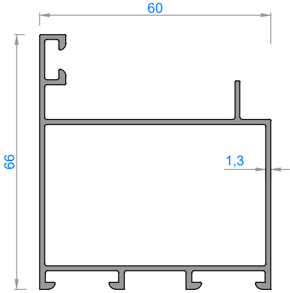
1157 - 0,975 kg/m
