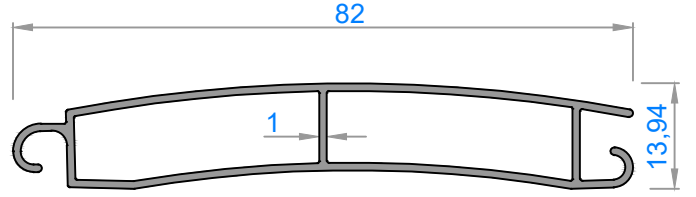
3254 - 0,532 kg/m
