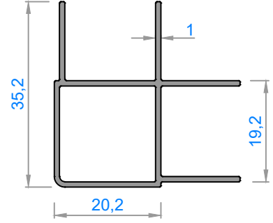
4798 - 0,369 kg/m
