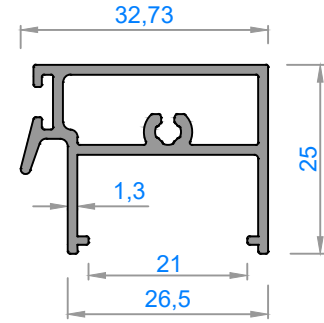
6206 - 0,455 kg/m
