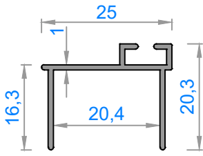
1206 - 0,187 kg/m
