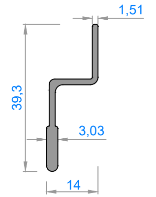
1142 - 0,257 kg/m
