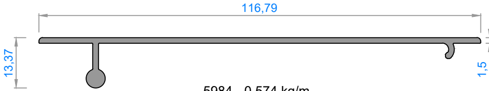
5984 - 0,574 kg/m
