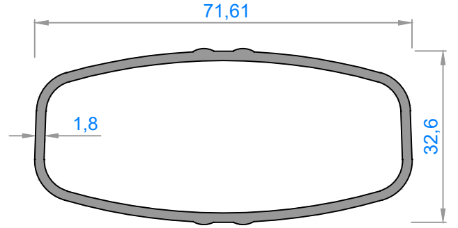
1511 - 0,865 kg/m
