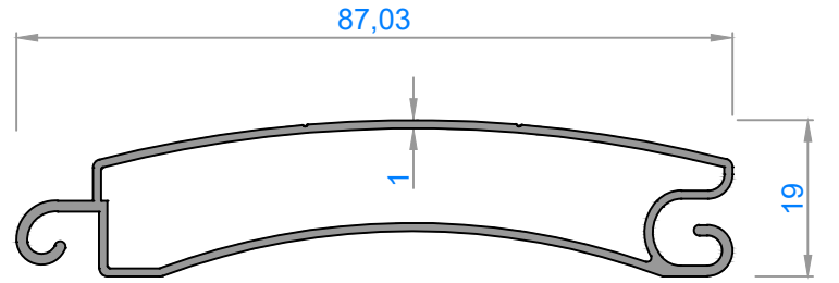
1505 - 0,607 kg/m
