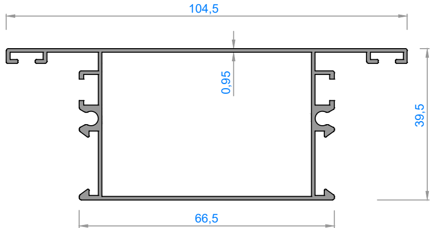
2598 - 0,848 kg/m
