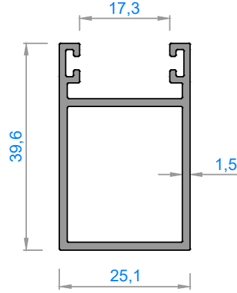
5123 - 0,541 kg/m
