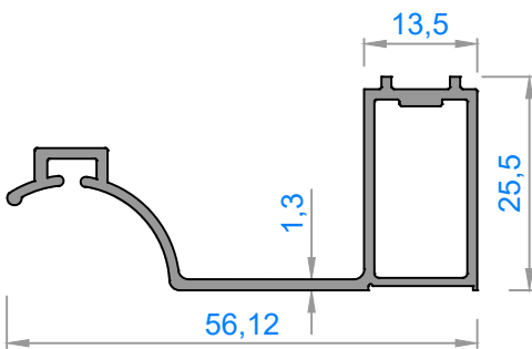
1285 - 0,455 kg/m STOK BOYU : 550 cm
