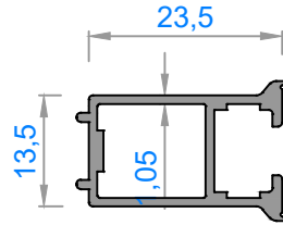
1286 - 0,269 kg/m STOK BOYU : 550 cm
