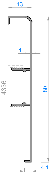
4345 - 0,355 kg/m
