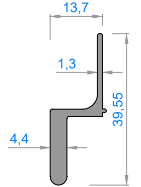
2099 - 0,359 kg/m
