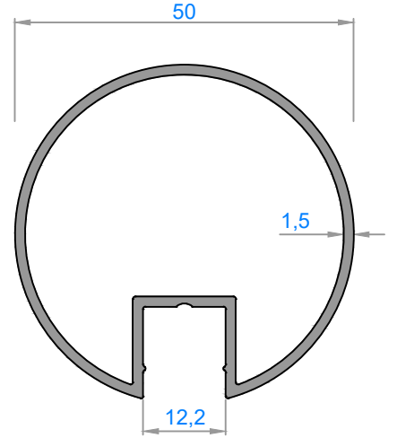
3761 - 0,726 kg/m
