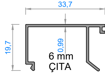
*4327 - 0,218 kg/m
