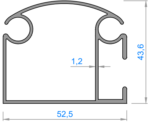
1190 - 0,791 kg/m
