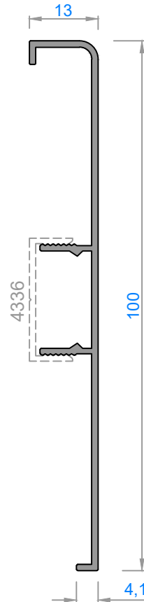
4347 - 0,445 kg/m
