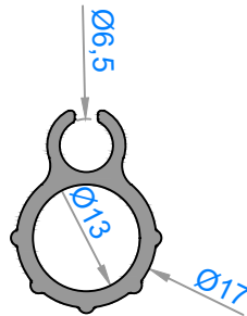
5126 - 0,340 kg/m
