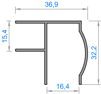
4401 - 0,363 kg/m
