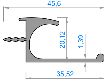
2508 - 0,428 kg/m
