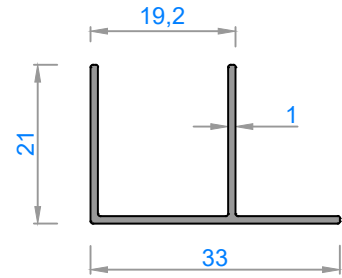
4795 - 0,197 kg/m
