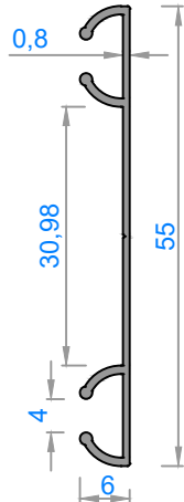
4408 - 0,191 kg/m
