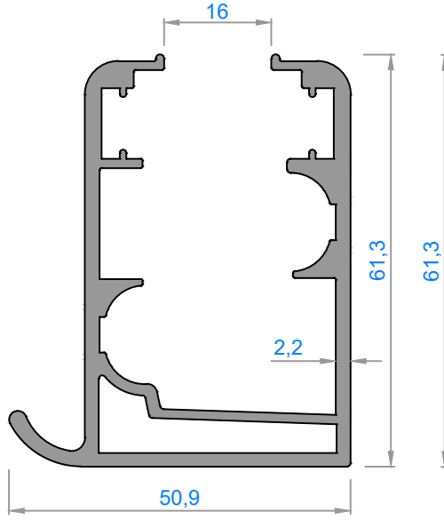
5297 - 1,496 kg/m
