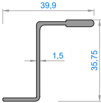
2448 - 0,345 kg/m
