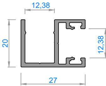
* 4337 - 0,370 kg/m
