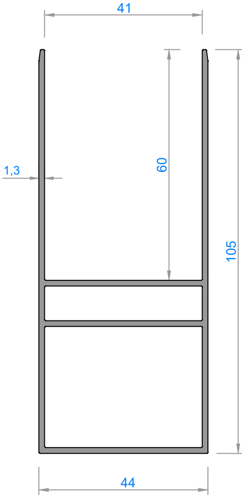
4185 - 1,175 kg/m
