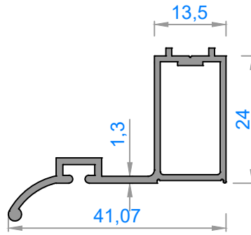
1281 - 0,380 kg/m STOK BOYU : 550 cm
