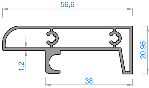
4797 - 0,661 kg/m
