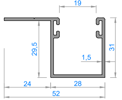
2317 - 0,531 kg/m
