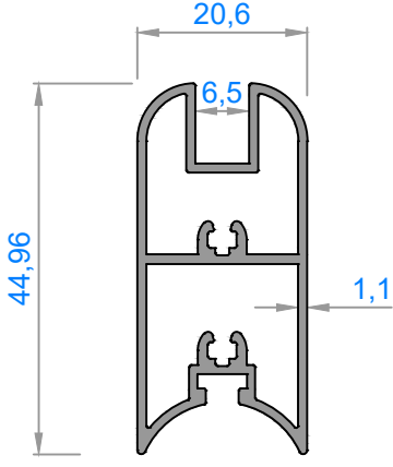
3390 - 0,579 kg/m
