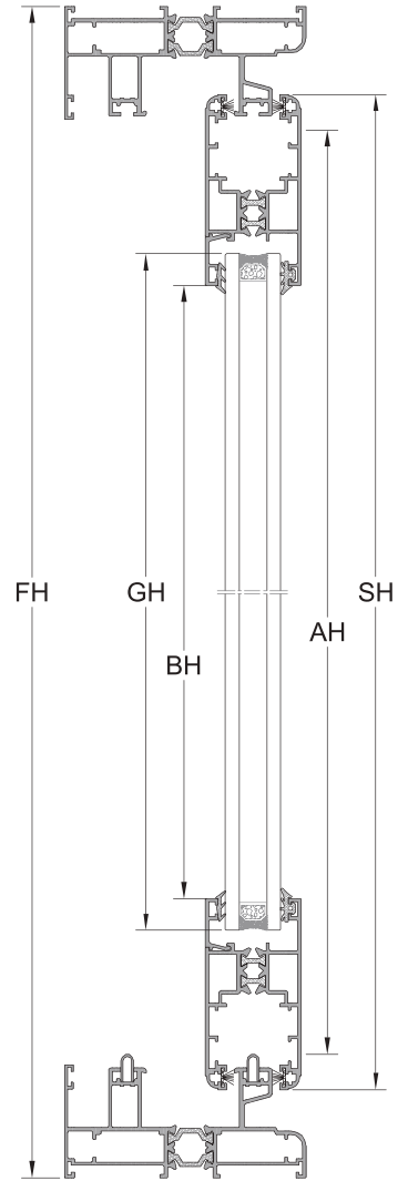
C-C KESİTİ
