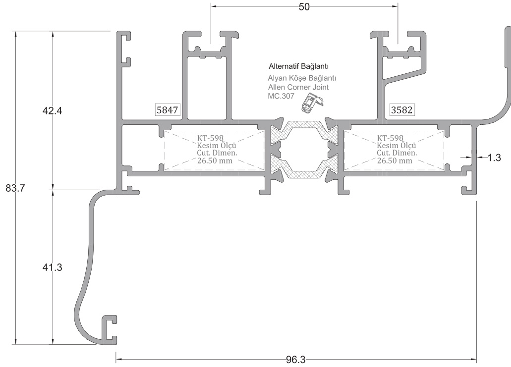
İki Raylı Sineklilikli Kasa Profili DOUBLE RAIL SCREENING FRAME PROFILE
