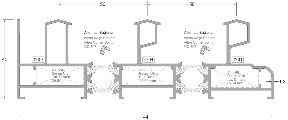
Üç Raylı Kasa Profili TRIPLE RAIL FRAME PROFILE
