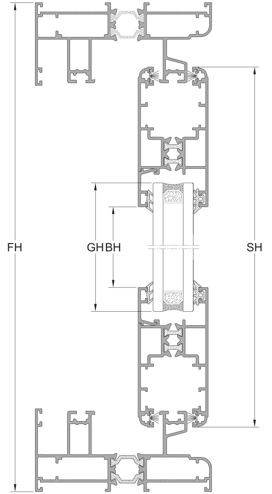
B-B KESİTİ
