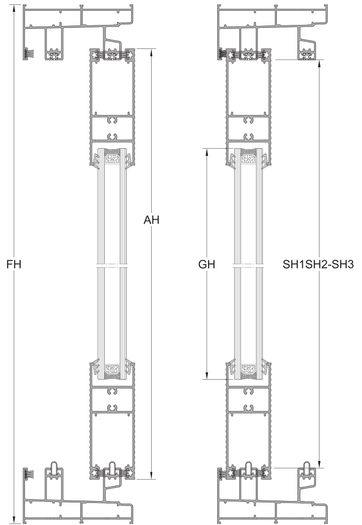
B-B KESİTİ
