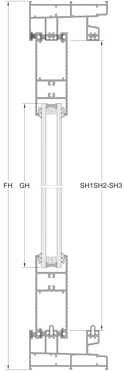
B-B KESİTİ
