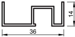
No : 825 0,280 kg/m
