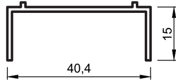
No : 3944 0,250 kg/m
